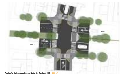
Diseño de Intersección en Norte 4 y Puente 117 - 100 m
